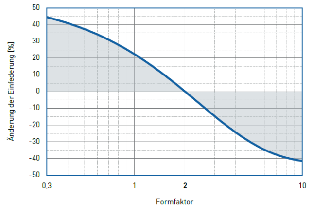
Einfederung
